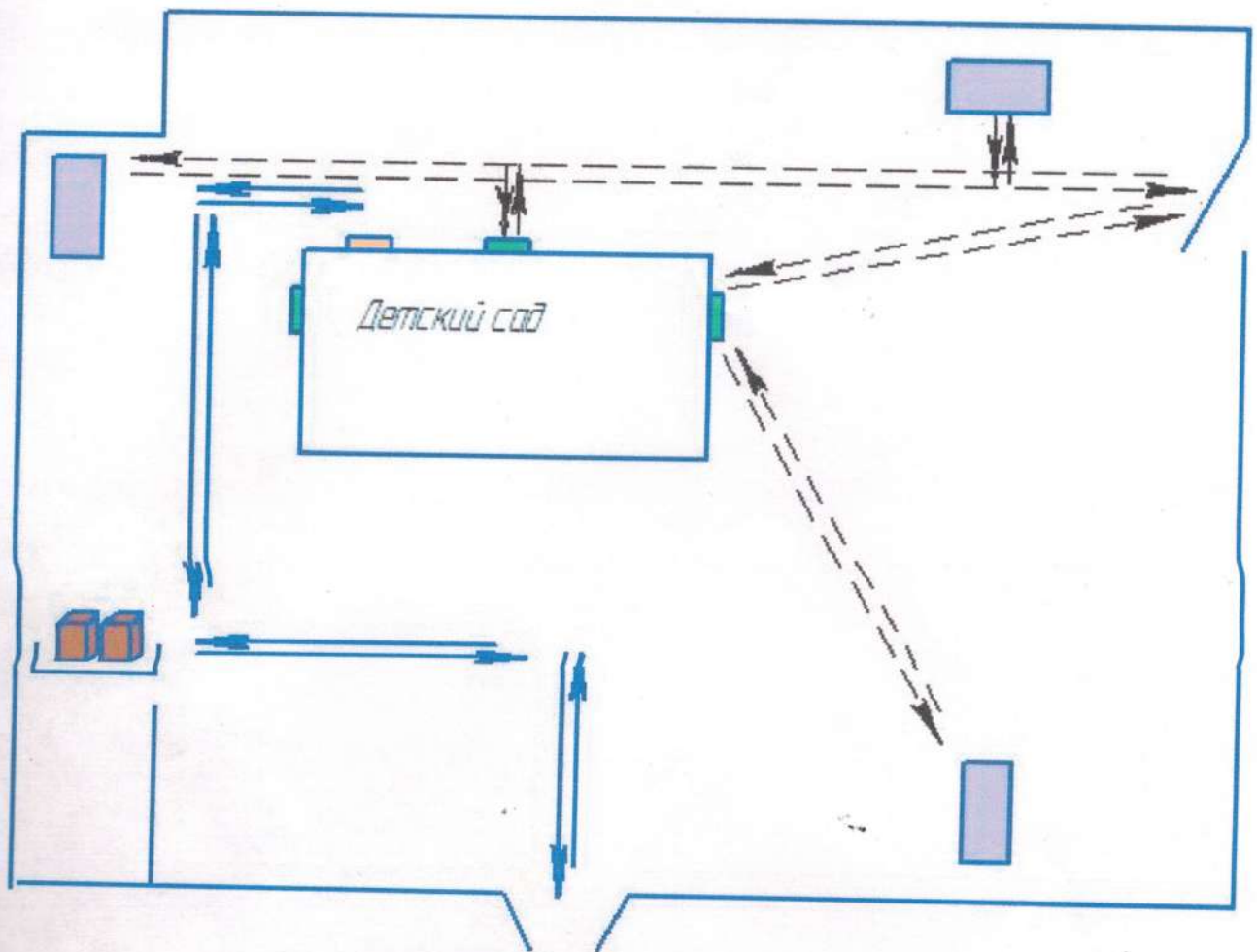
Схема 3. Пути движения транспортных средств к местам разгрузки/погрузки и рекомендуемые безопасные пути передвижения детей по территории дошкольной образовательной организации.
